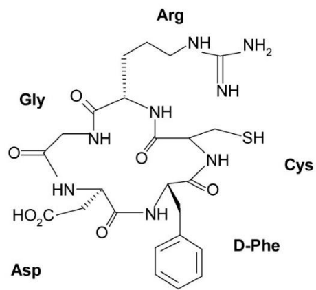
ciklo[RGDfC]
