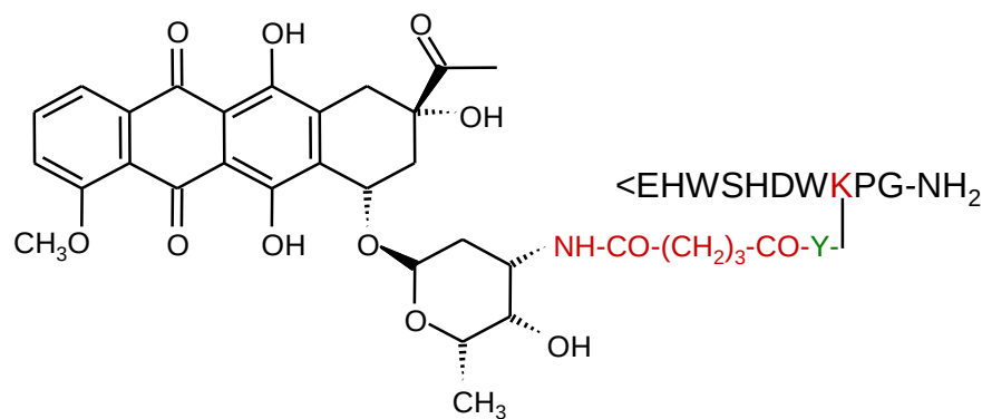
amid-kötés
