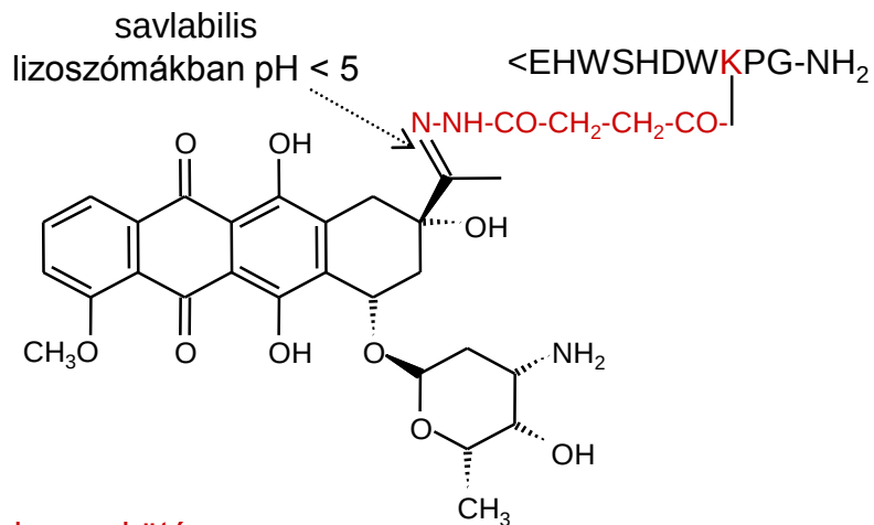
hidrazon-kötés
