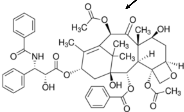
paclitaxel
